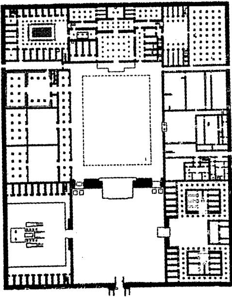
٣٥ قصر كل من الملك إخناتون بتل العمارنة ومرنبتاح بمنف - دولة حديثة
